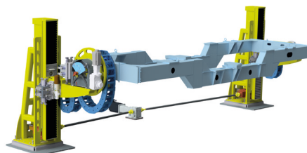
Hub-Dreheinheiten
