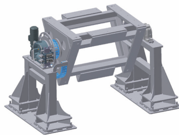
Posicionador de Giro sobre cavaletes
