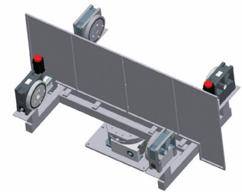
Posicionador de Giro célula 3 eixos H-Frame
