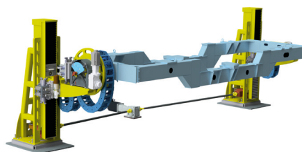
Posicionador de Elevação
