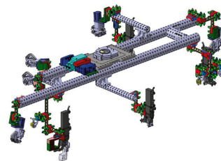
Garra de Manipulação de Robô Eurogreifer
