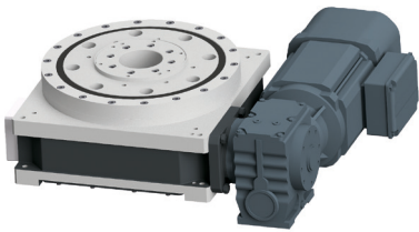
Mesas giratórias indexadoras RTX de divisões fixas
