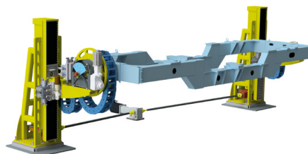
Unité de levage et rotation
