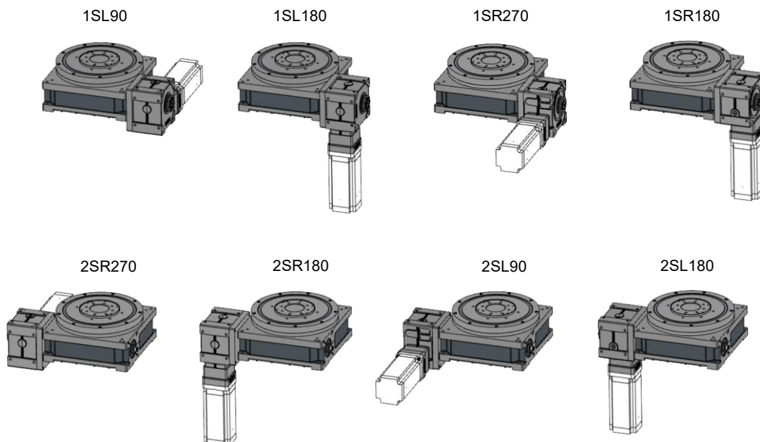
Abb. 8: Anbautagen Antrieb RTF
