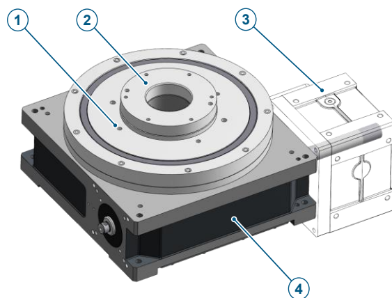
Abb. 4: Aufbau Trommelkurvenrundtisch – Distanzausführung
