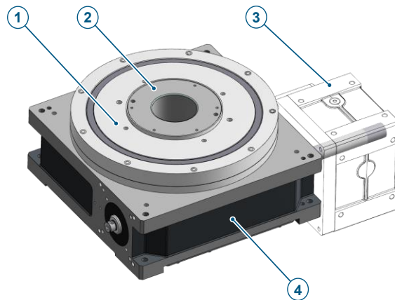
Abb. 3: Aufbau Trommelkurvenrundtisch – Basisausführung
