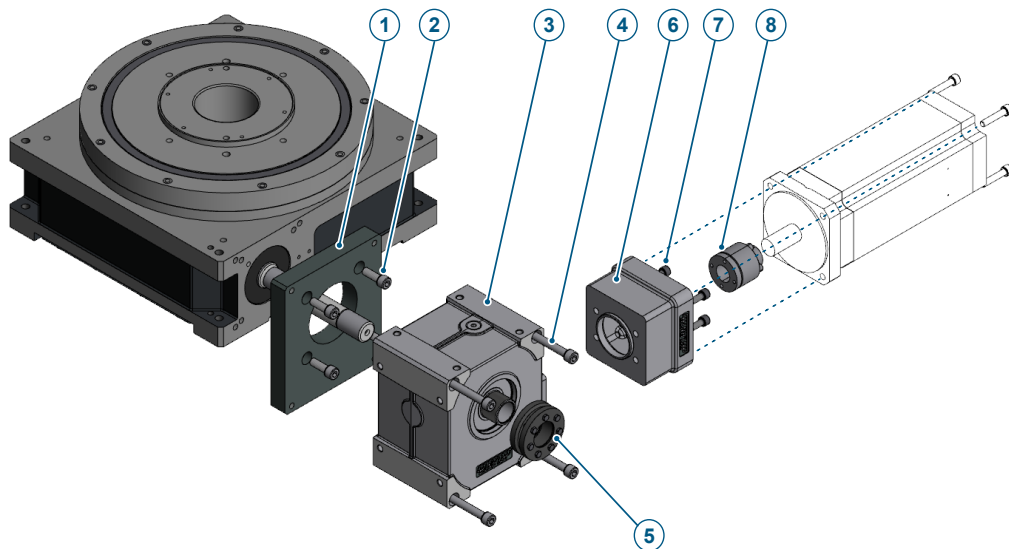
Abb. 9: Anbaureihenfolge Antrieb
